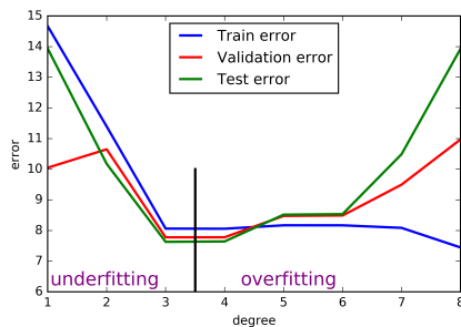
Hình 1: Overfit & Underfit
